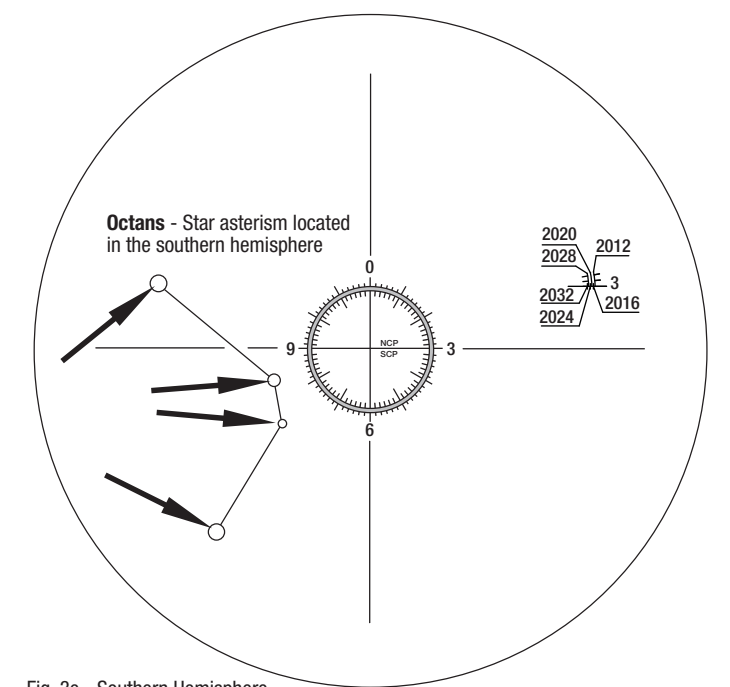
Fig. 3e - Southern Hemisphere
